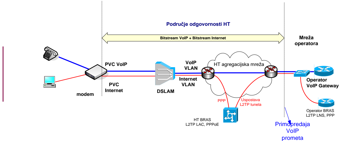
Slika 12. Realizacija posebnog virtualnog kanala za VoIP uslugu preko ADSL/VDSL pristupa (kod VDSL pristupa između modema i DSLAM-a koristi se odgovarajući VLAN)
